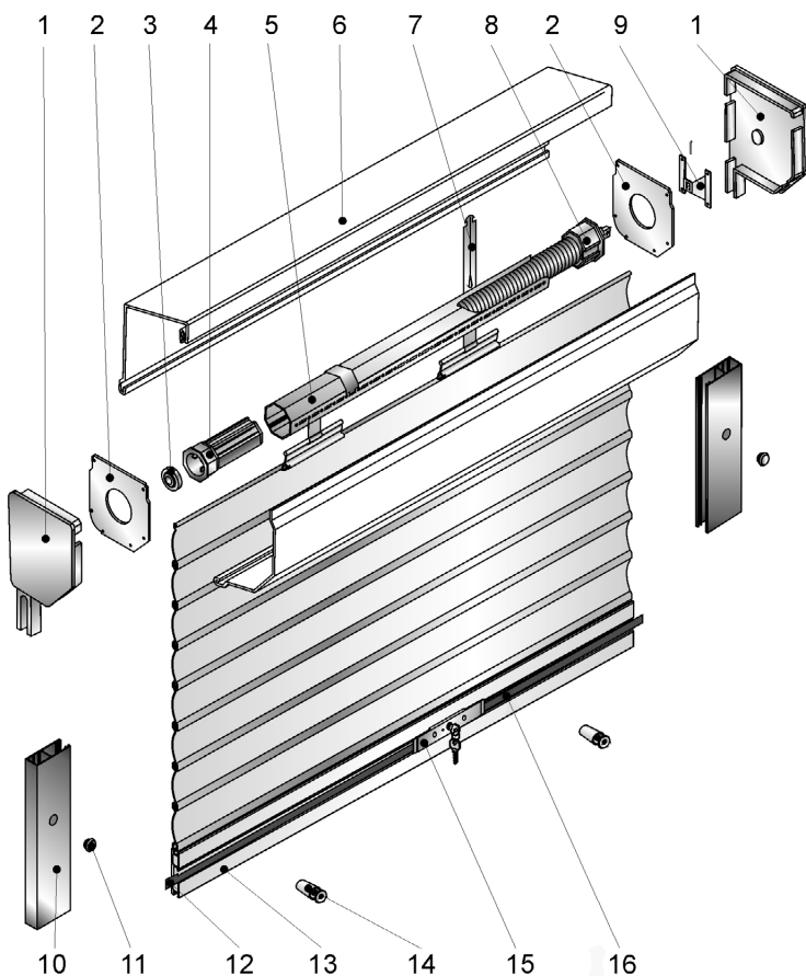
Рис. 6. Комплектация роллет со шнуровым или кордовым приводом:
